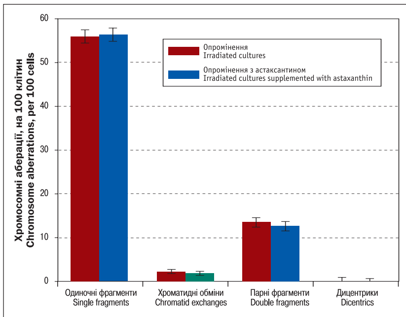
Рисунок 1. Спектри аберацій хромосом в опроміненіх на G 2 стадії клітинного циклу культурах лімфоцитів периферичної крові людини та в опроміненіх культурах при додаванні астаξανтину.
